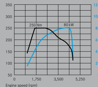
A 180 CDI
